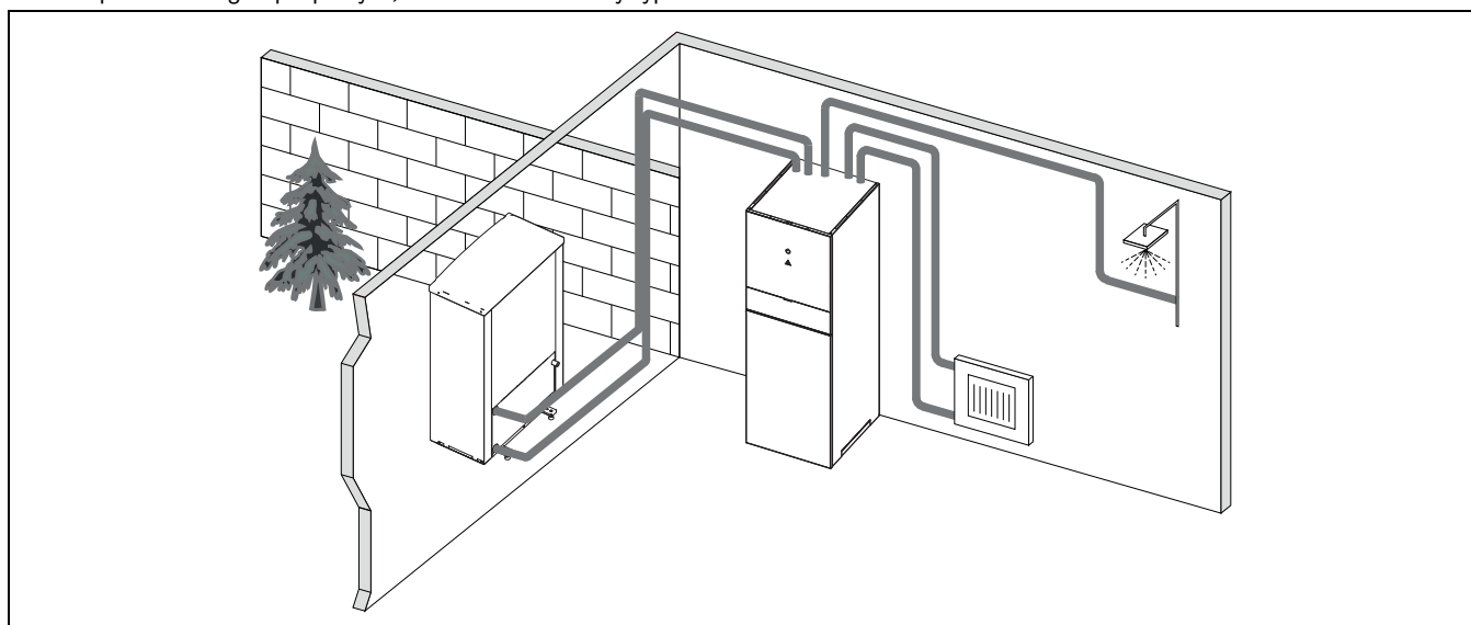
Obr. 3 Tepelné čerpadlo AirX 400, vnitřní jednotka AirModule E / AirModule S/W s integrovaným zásobníkem teplé vody a elektrickou pomocnou topnou tyčí
