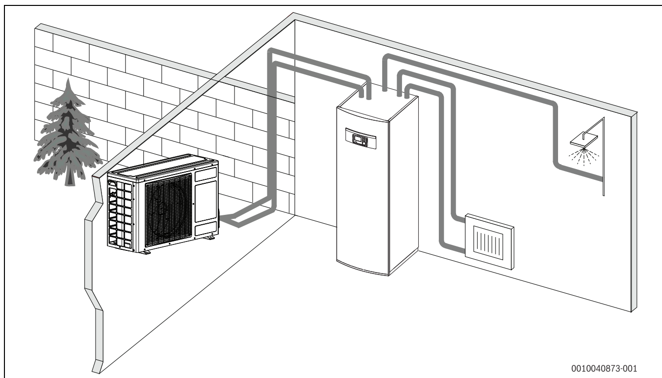
Obr. 2 Tepelné čerpadlo pro venkovní jednotku, vnitřní jednotku AirModule Split s integrovaným zařízením na přípravu teplé vody a elektrickou pomocnou topnou tyčí
