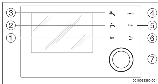
Obr. 3 Ovládací prvky
