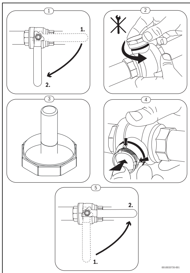
Obr. 5 Čištění sítka
